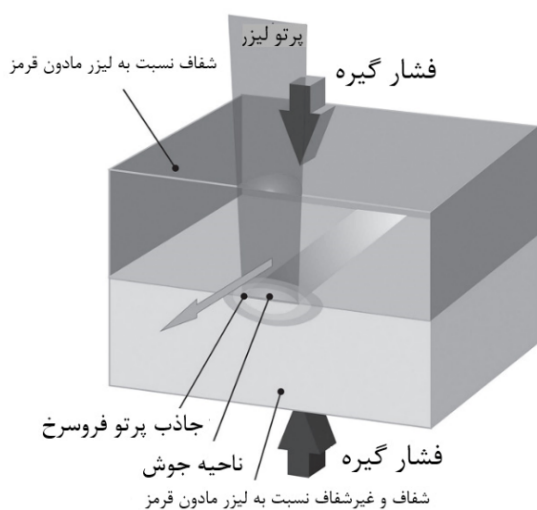
شکل ۱: نمای شماتیکی از فرایند جوشکاری لیزر عبوری [۴]
