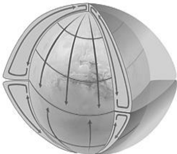
شکل ۲ جریان هوا در صورت عدم چرخش زمین به دور خود [۱۳]
