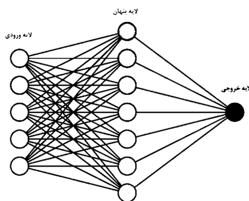
شکل ۱. شبکه عصبی با یک لایه پنهان
