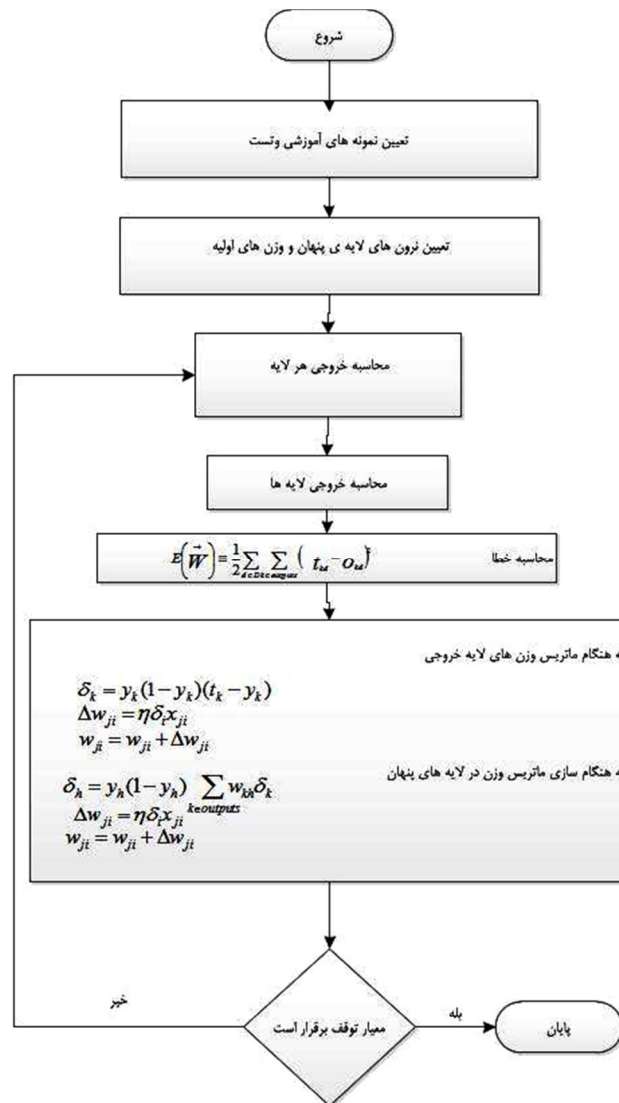
شکل ۲. فلوجارت شبکه عصبی پرسپترون با الگوریتم پس انتشار خطا
